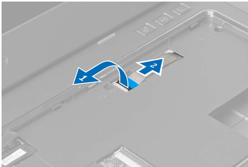
7. ถลายสกรู จากนั้นปลดสาย LVDS ออกจากเมนบอร์ด
